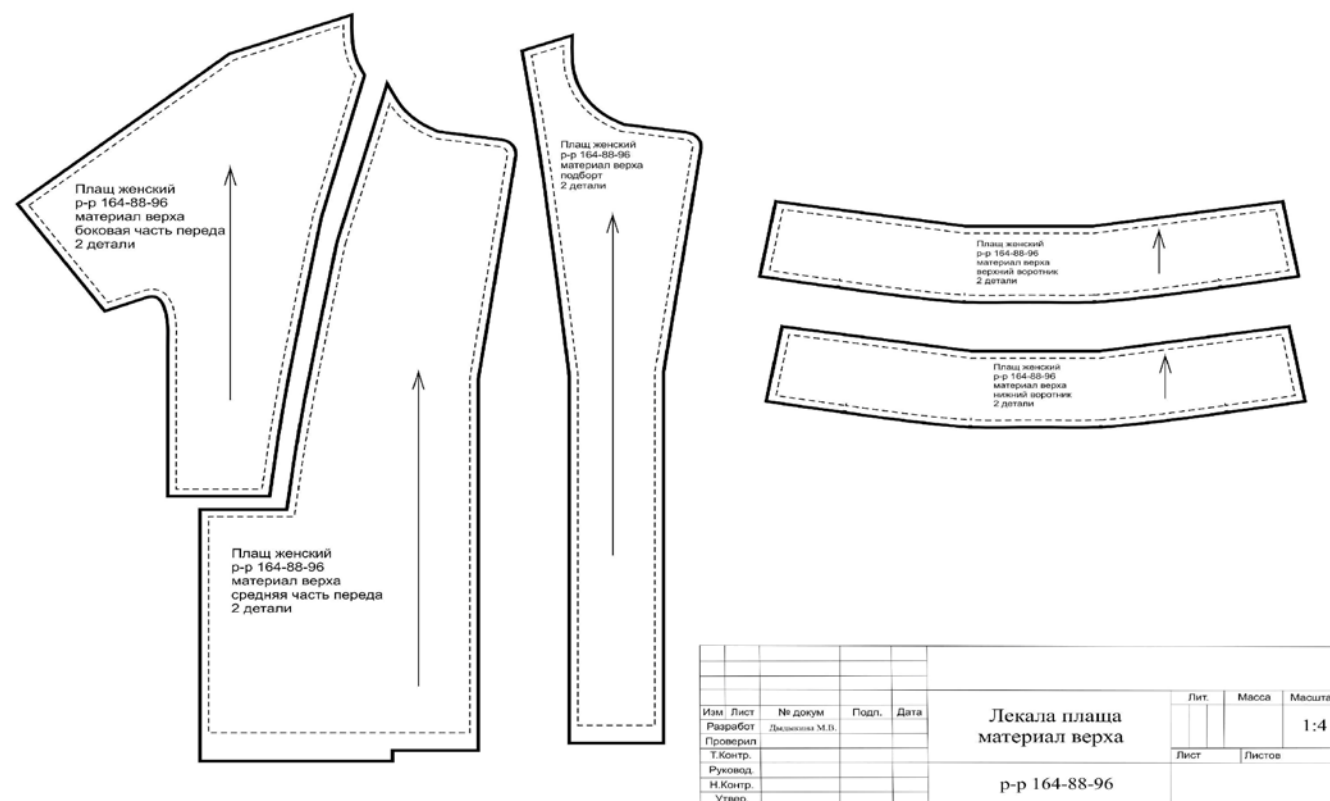
Рисунок 12.1 Пример оформления лекал
