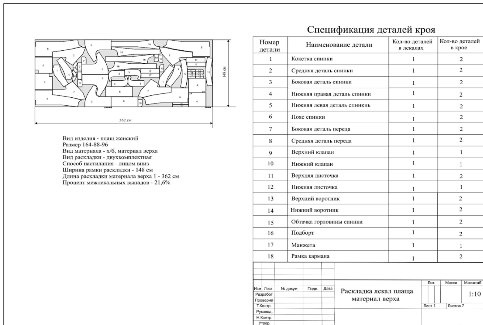
Рисунок 12.2 Пример оформления раскладки лекал
